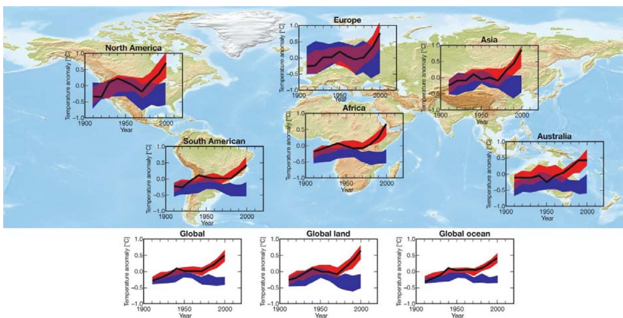
Abbildung 3: Beobachtete Temperaturentwicklung auf dem Globus und verschiedenen Gebieten (schwarz), sowie Ensembles der Temperaturentwicklung mit Modellen, die entweder nur natürliche Faktoren (blau) oder nur anthropogene Faktoren (rot) berücksichtigen. (IPCC, 2007)
