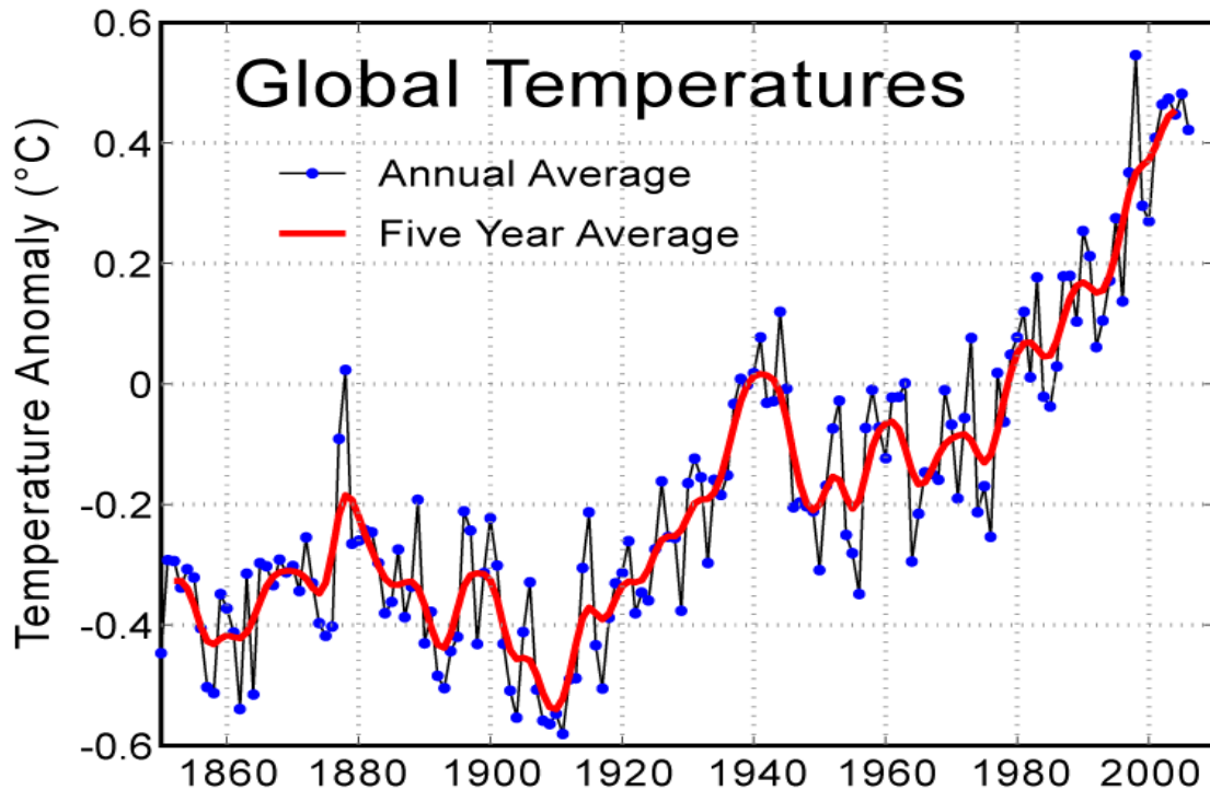
Abbildung 1: Entwicklung der global gemittelten Temperatur der Luft bis 2007. (Zoirta, pers. Mitt.)
